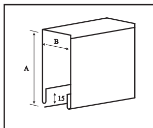
krycí plech typ (KP 3) rozvinutá šířka = (2 \cdot A) + B
