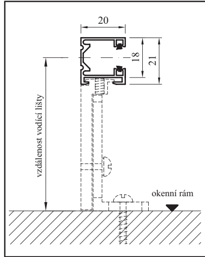
Vodící lišta typ 2 - jednoduchá (VL 2)
