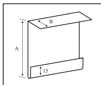
krycí plech typ 1 (KP1)
