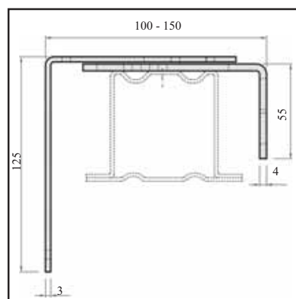
Držák krycího plechu typ 5 (DK 5)
