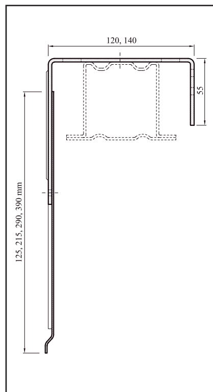
Nástavec s držákem krycího plechu
