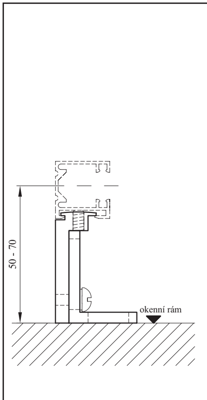
Konzola vodící lišty - K 1
