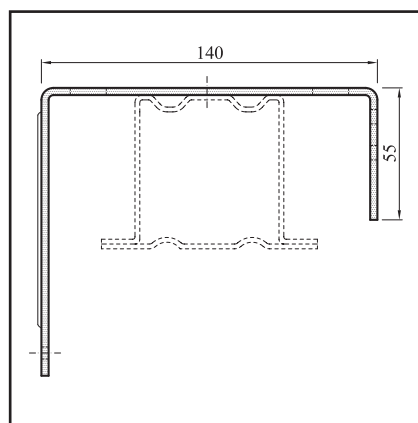
Držák krycího plechu typ 4 pro Z-90 (DK 4)
