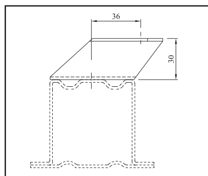
„Z“ držák pro F-80 do překladu HELUZ - příčný řez
