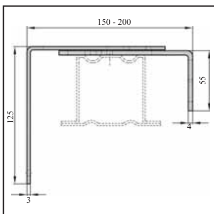
Držák krycího plechu typ 6 (DK 6)
