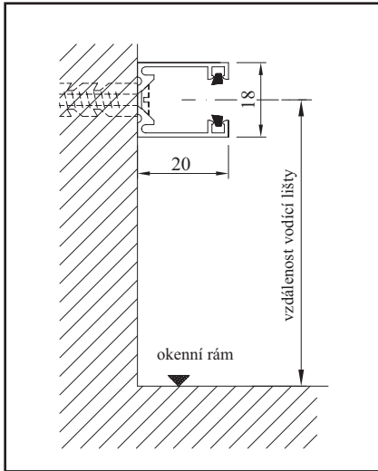
Vodící lišta typ 1 - do ostění (VL 1)
