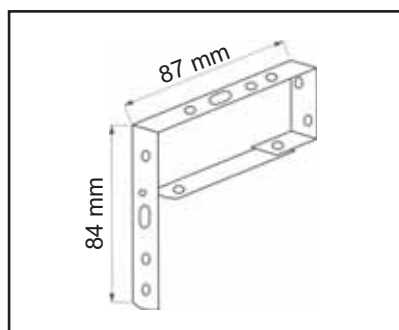
- držák krycího plechu (na zeď i strop)
