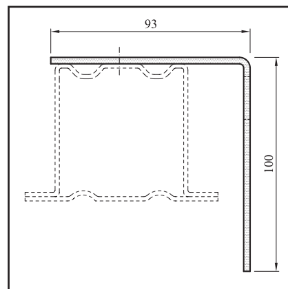
Montážní držák typ 2b - montáž na stěnu (MD 2b)
