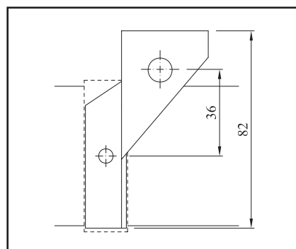
„Z“ držák pro F-80 do překladu HELUZ - půdorys
