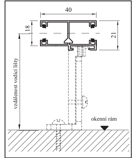
Vodící lišta typ 3 - dvojitá (VL 3)
