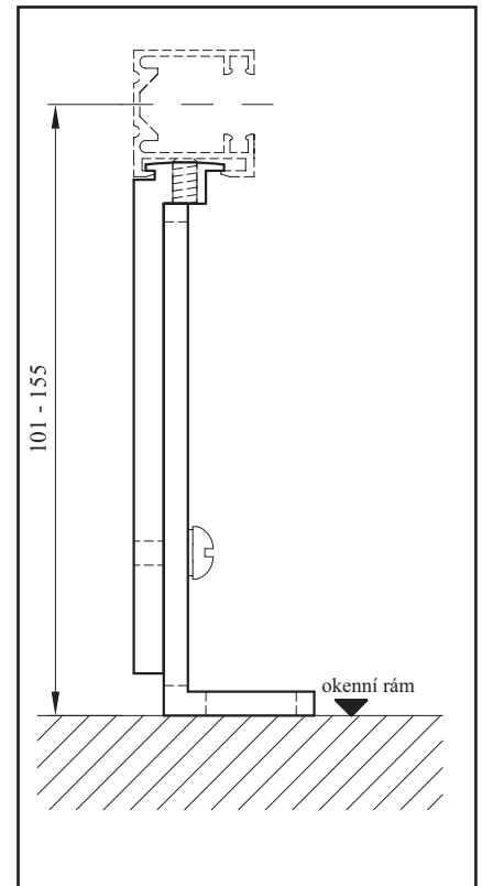
Konzola vodící lišty - K 3
