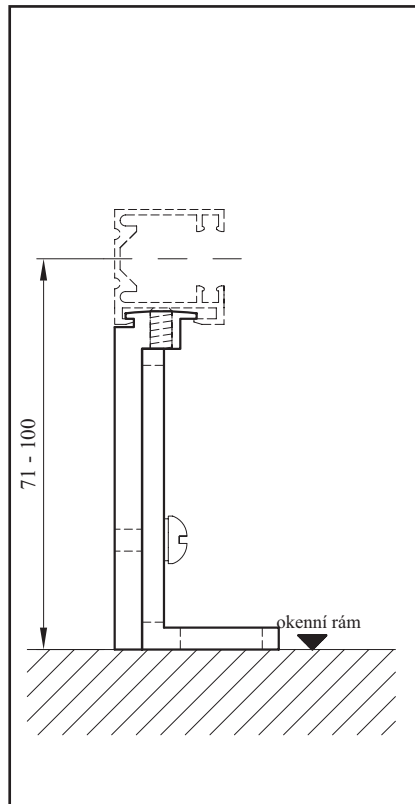
Konzola vodící lišty - K 2
