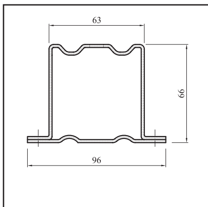
Montážní držák typ 1 - samostatný (MD 1)
