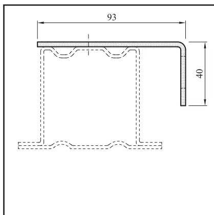
Montážní držák typ 2a - montáž na stěnu (MD 2a)
