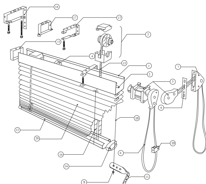
Popis komponentů venkovní žaluzie EXT-50 Obrázek č. 39
