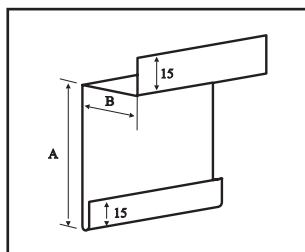
krycí plech typ 2 (KP 2)
