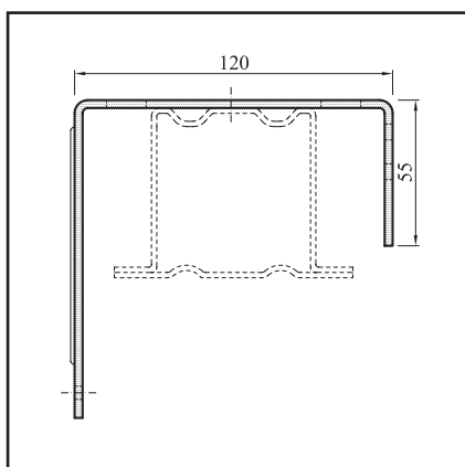
Držák krycího plechu typ 3 pro C-80, F-80 (DK 3)
